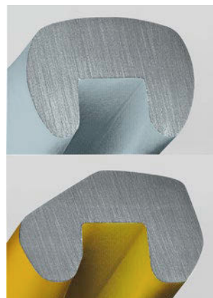
Comparación de la sección transversal del rebaje de una aguja estándar (arriba) y una aguja SAN® 6 GEBEDUR® (abajo)
